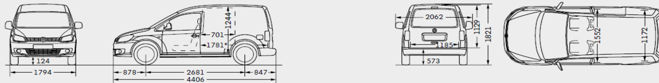
Caddy Bestelwagen EcoFuel
