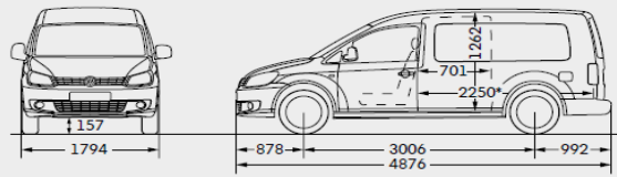
Caddy Maxi Bestelwagen
