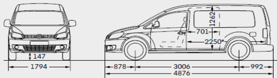
Caddy Maxi Bestelwagen EcoFuel
