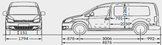
Caddy Maxi Bestelwagen 4MOTION
